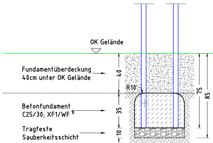
FUNDAMENTSCHNITT(E) M 1:20
