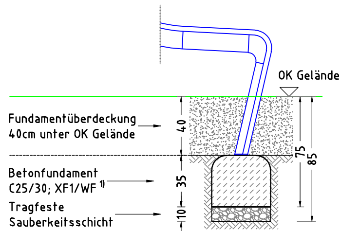
FUNDAMENTSCHNITT(E) M 1:25
