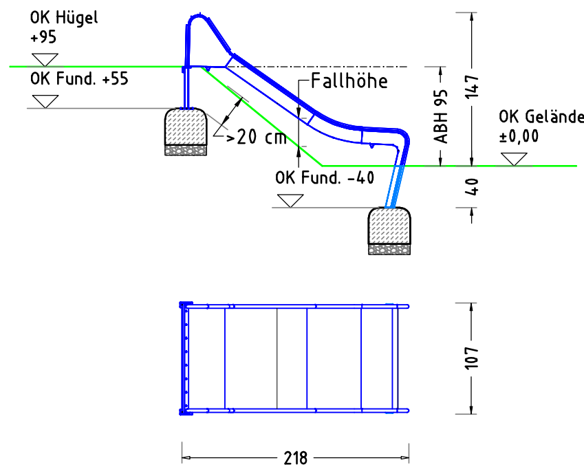
GELÄNDESCHNITT M 1:50
