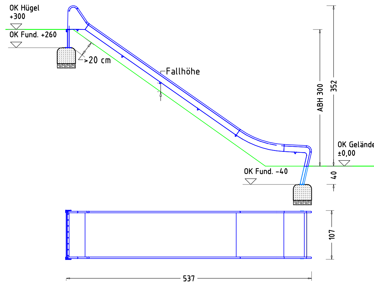
GELÄNDESCHNITT M 1:50
