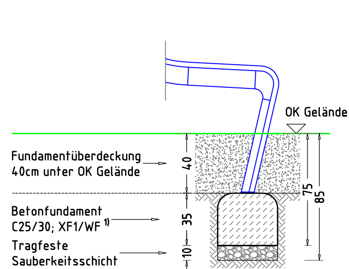
FUNDAMENTSCHNITT(E) M 1:25
