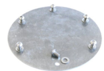
EME-Z-6150 Montageflansch- abdeckung als Winterschutz
