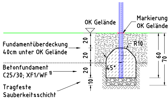
FUNDAMENTSCHNITT(E) M 1:25
