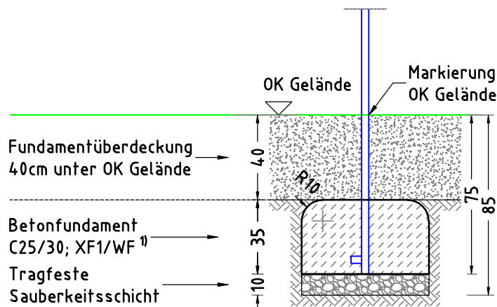
FUNDAMENTSCHNITT(E) M 1:25
