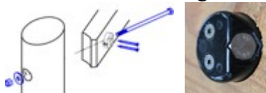
Geländerverschraubung
