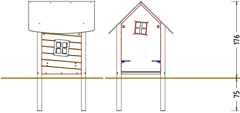
Giebelverkleidung mit Fenster
