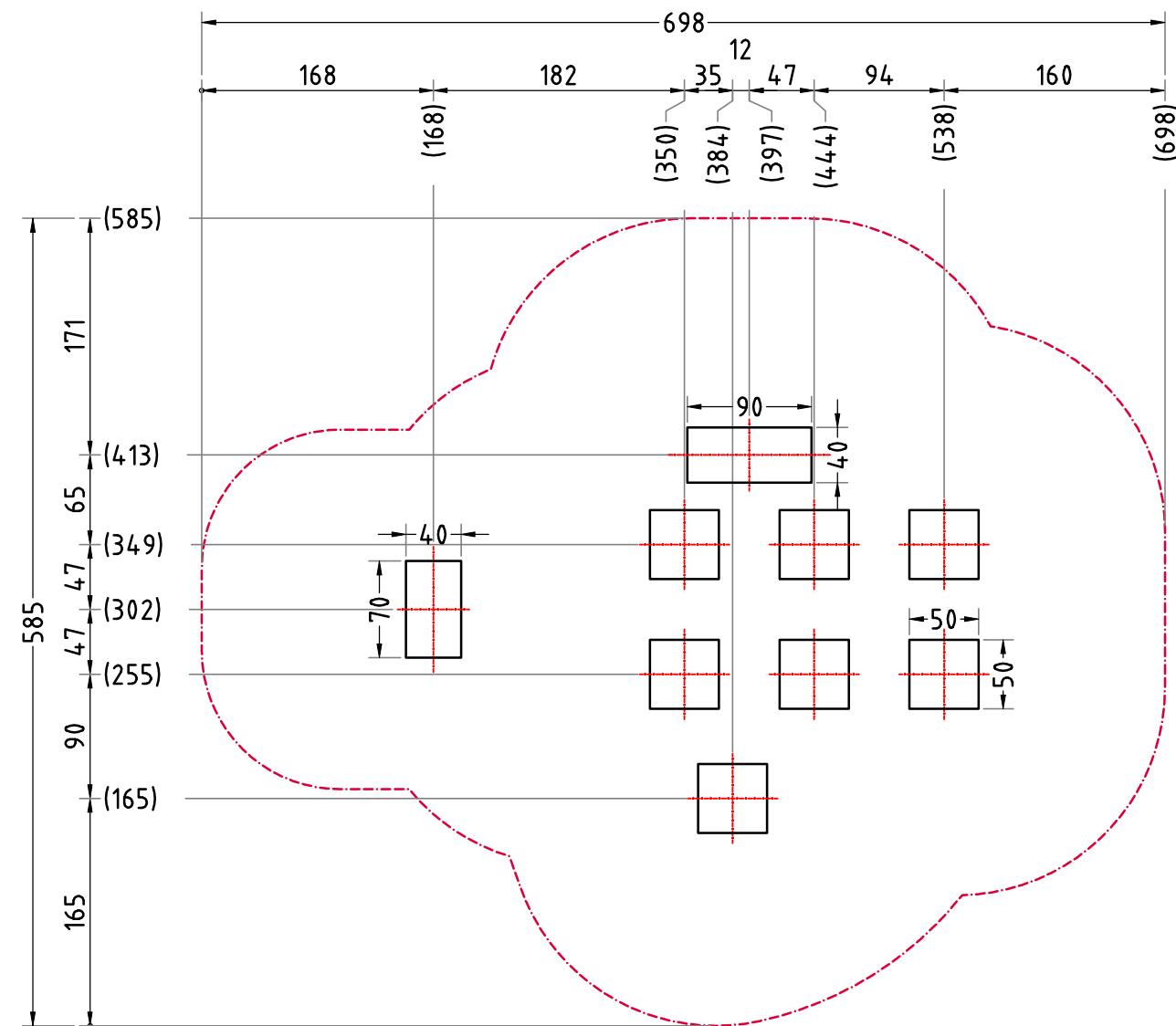
FUNDAMENTSCHNITT(E) M 1:25
