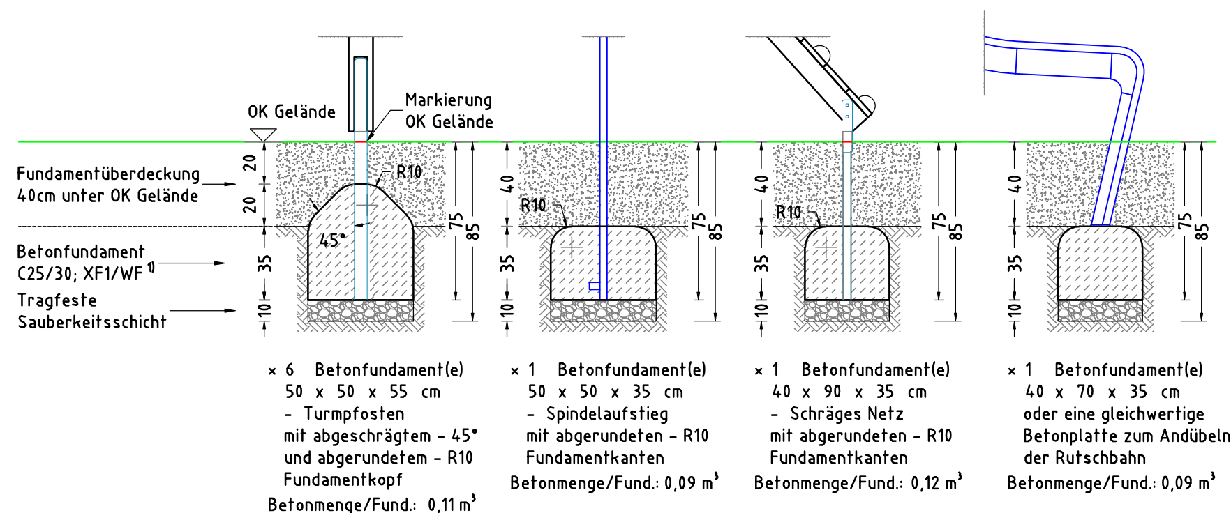
FUNDAMENTSCHNITT(E) M 1:25
