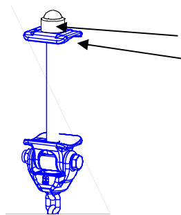
Abdeckkappe Gegenplatte
