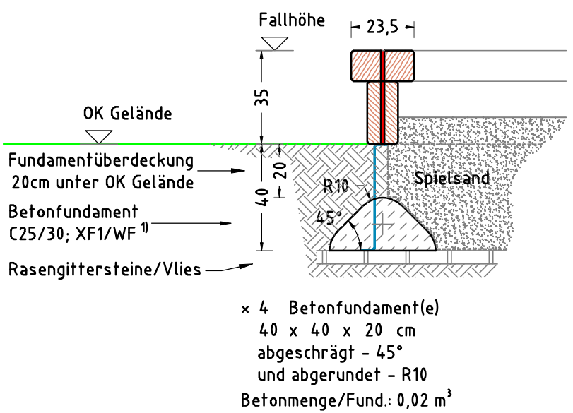
FUNDAMENTSCHNITT(E) M 1:20
