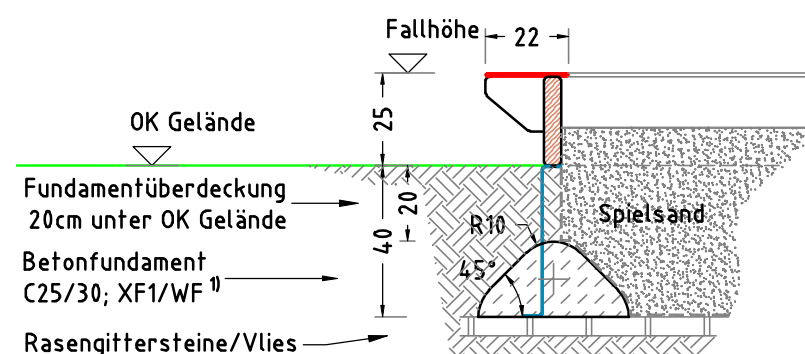
FUNDAMENTSCHNITT(E) M 1:20
