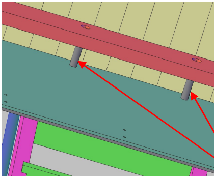
Kunststoff - Rohr zwischen Ebene und HPL-Platte
