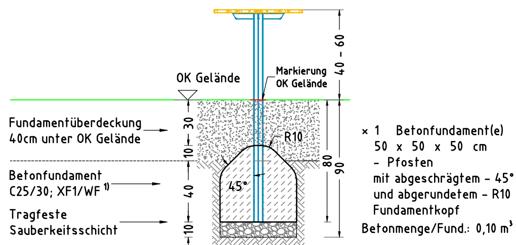
FUNDAMENTSCHNITT(E) M 1:25
