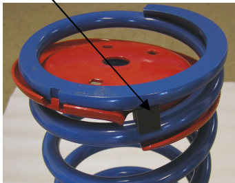
Muttern an den Federtellern (Drehmoment 30Nm)
