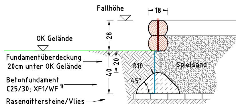
FUNDAMENTSCHNITT(E) M 1:20
