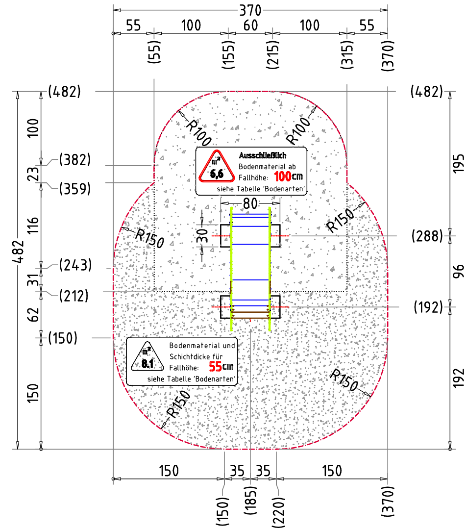
FUNDAMENTSCHNITT(E) M 1:20
