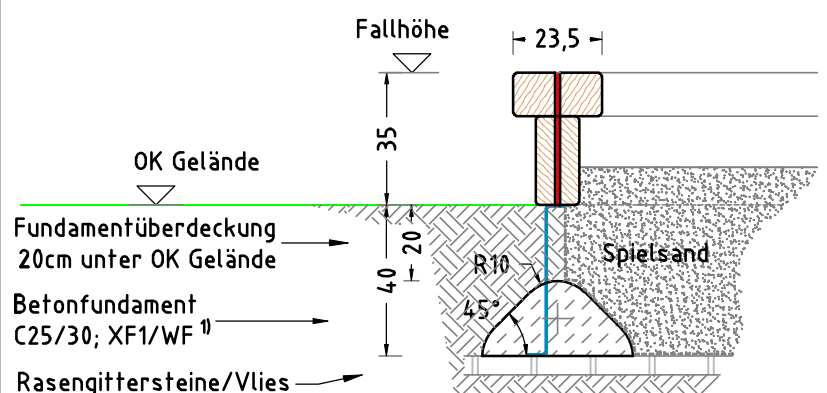
FUNDAMENTSCHNITT(E) M 1:20
